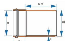
TUBO PVC COLETOR DE ESGOTO OCRE COM JUNTA ELÁSTICA INTEGRADA - PRESSURIZADO PN16 (CONFORME ABNT NBR 7665)
