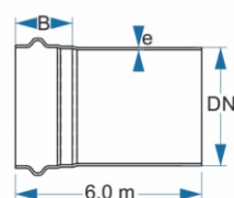
TUBO PVC PARA ESGOTO SANITÁRIO - SN (SÉRIE NORMAL) (CONFORME ABNT NBR 5688:1999)
