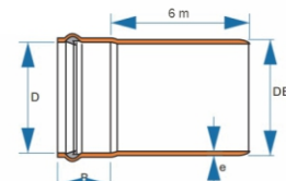
TUBO PVC COLETOR DE ESGOTO OCRE COM JUNTA ELÁSTICA INTEGRADA - PRESSURIZADO PN10 (CONFORME ABNT NBR 7665)
